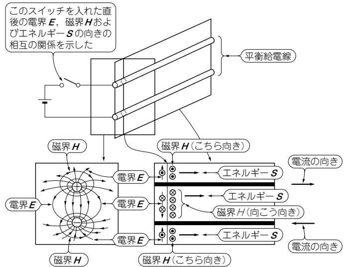
図5-2 平衡給電線に電圧をかけた直後の 電界、磁界、エネルギーの方向
