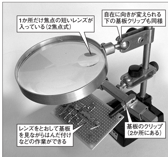
写真10-1 基板ホルダー付きルーペ
