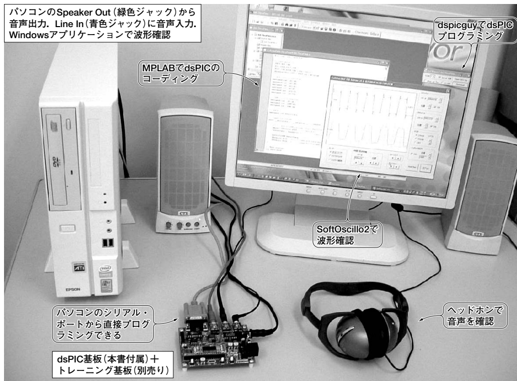
写真1 dsPICを使ったデジタル信号処理の実験風景。パソコン1台あれば実験できる！
