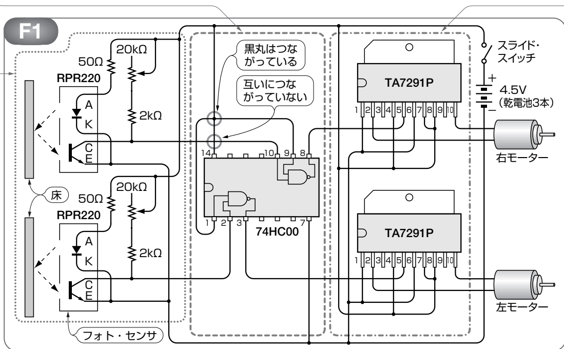
基本形のライトレース・カーの回路図(破線で囲った部分が、各基板に対応している。ロジック IC とモーター制御用 IC は、実物を上から見た図。ただしロジック IC の実物には \square の記号は記入されていない)
