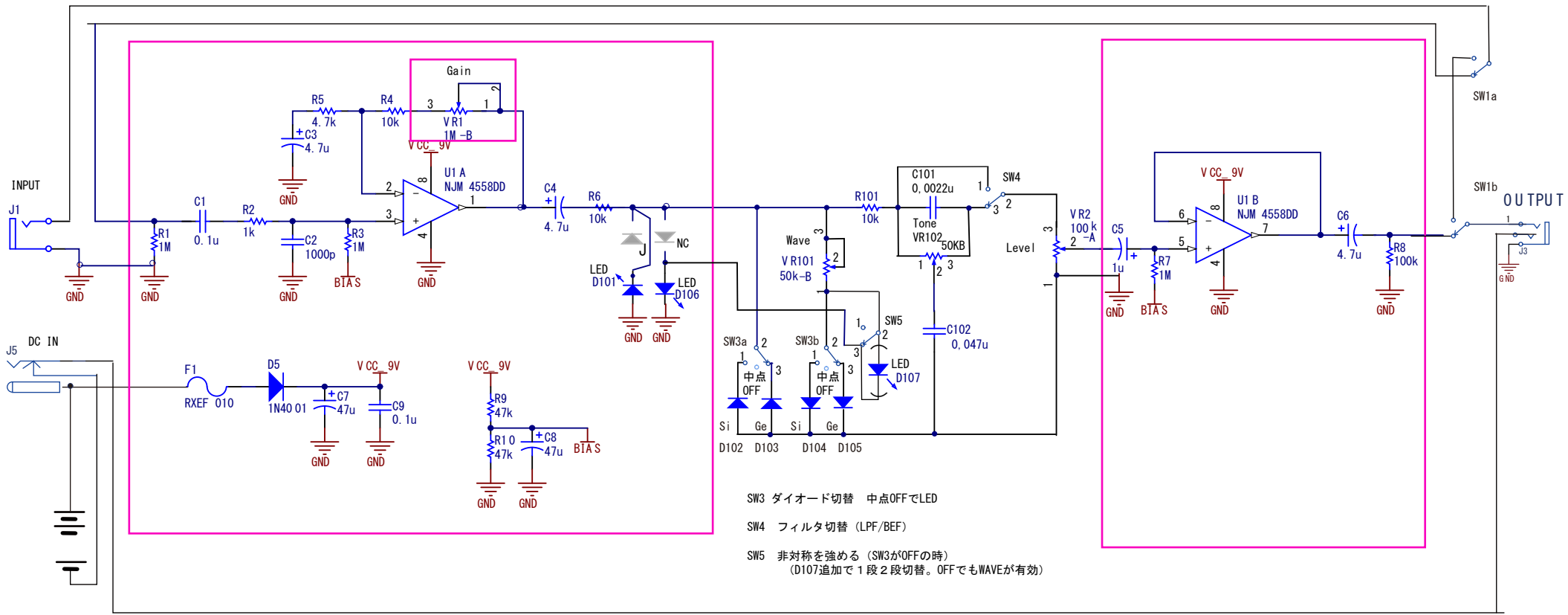
実用型組立 (本誌P43, 図1(a)+(b)に相当) D107追加は本誌出稿後の改良。
