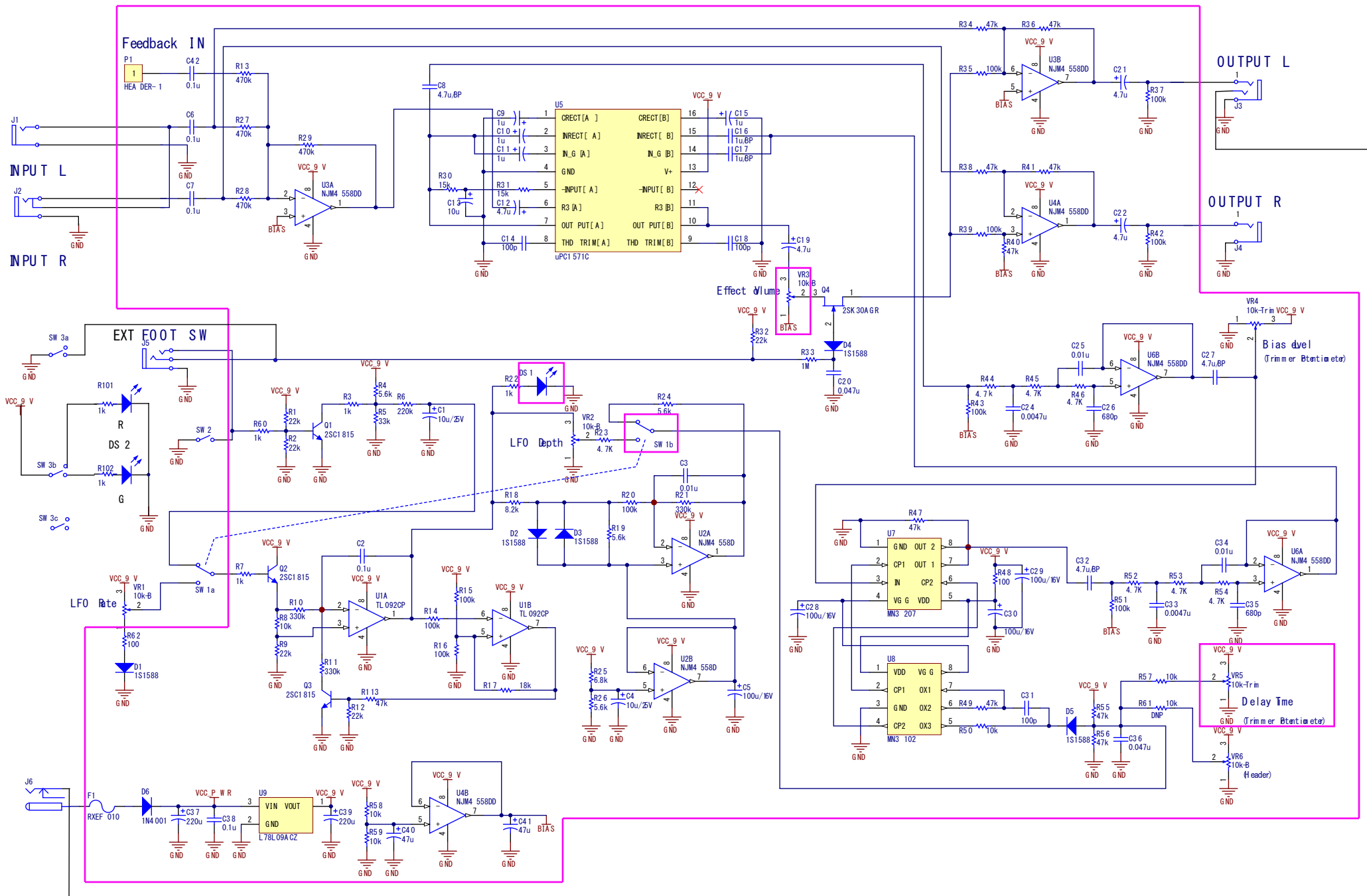
トラ技コーラスキット 電子スイッチでパスの配線
