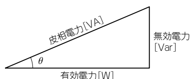
〈図3〉交流電力と力率 \cos \theta の関係
