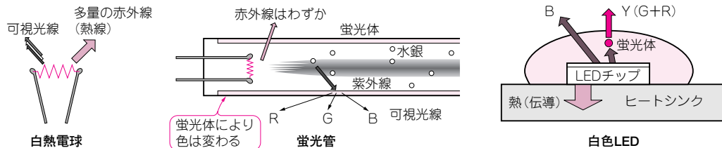
(b) 各種照明光源の構造
