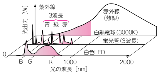
(a) 各種照明光源のスペクトル
