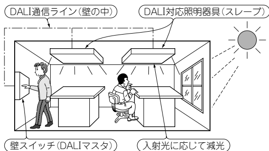
〈図1〉 DALI 対応照明器具を使った例
