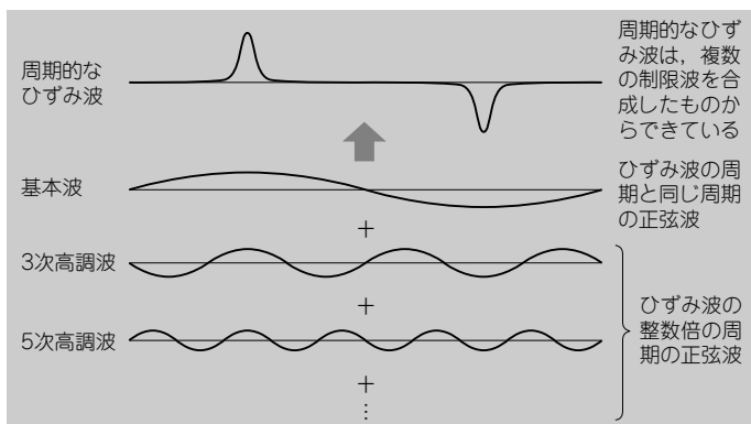
〈図2〉高調波の波形例 (1)
