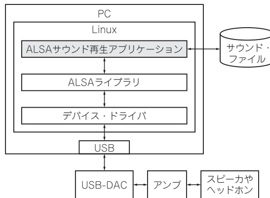
図1-6 PCオーディオ・システムの基本構成 USBインターフェース経由で高性能のD-A変換器を持つUSB-DACに接続する
